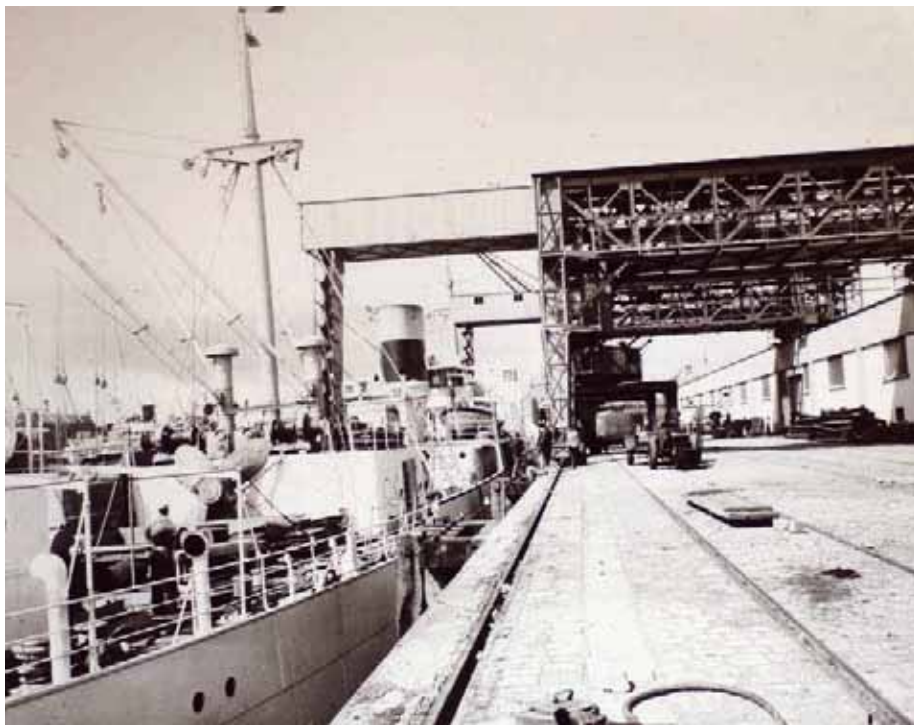
Sur le quai, les norias (tapis roulants à godets) descendaient vides dans la cale du navire et remontaient pleines de balles de bananes qui étaient acheminées vers le hangar.
